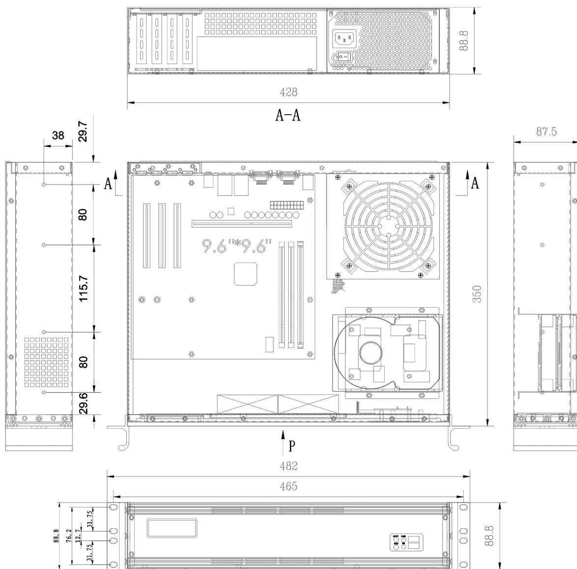
视图P
